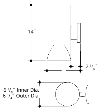
VW - WALL MOUNT
