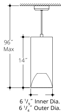
VP - PENDANT MOUNT
